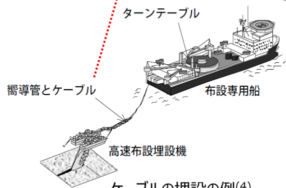
ケーブルの埋設の例(4)
