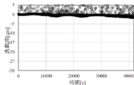
Case3 (洗掘防止工あり)
