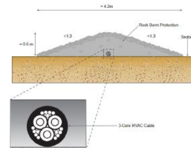
ケーブルを被覆した場合の断面(3)
