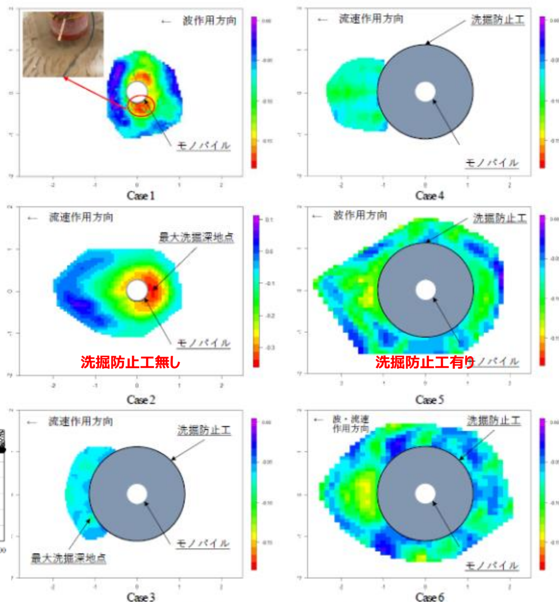
図-5 各ケースの最終洗掘深図 (単位: m)
