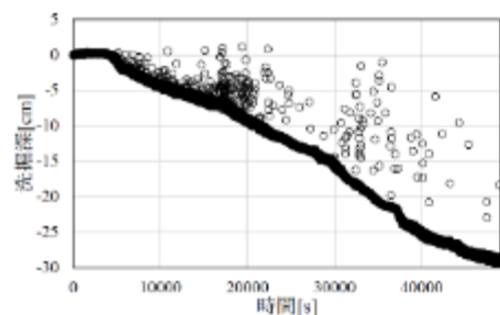
Case2 (洗掘防止工無し)
