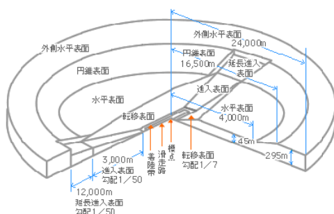
図 3.2.6-1 制限表面概略図
