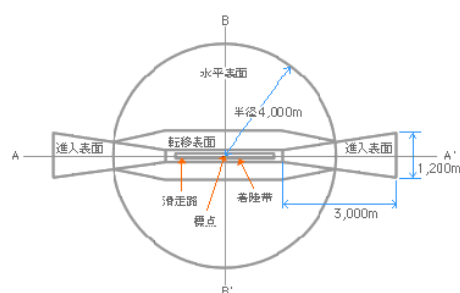
図 3.2.6-2 制限表面の平面概略
