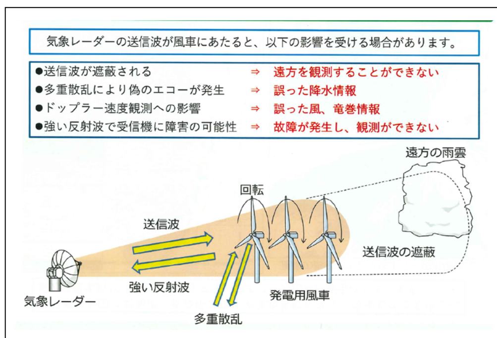
図 3.2.6-4 風車が気象レーダーへの及ぼす影響
