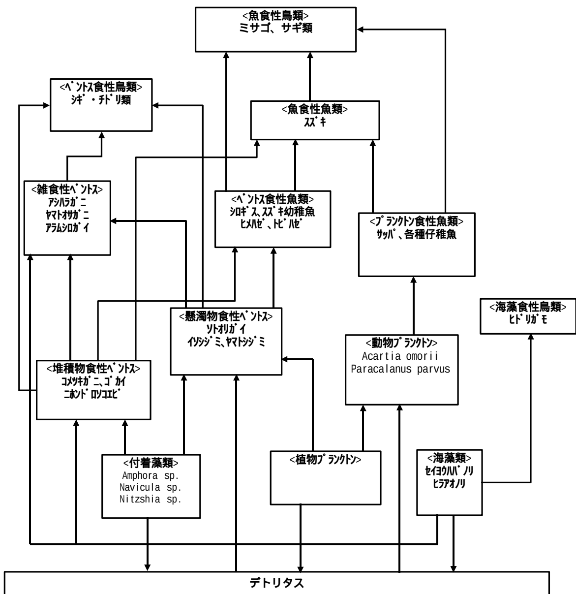
図 - 2.6 骨格的食物連鎖模式図 (例：汽水域の水中～水際)
