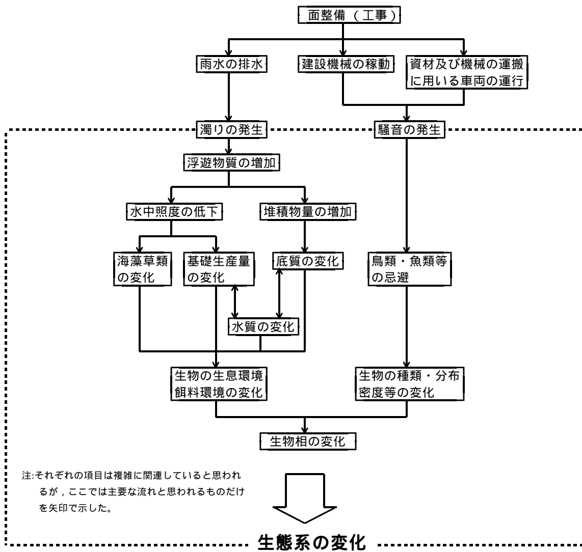
図 5 - 9 面整備の工事に係る環境影響フロー
