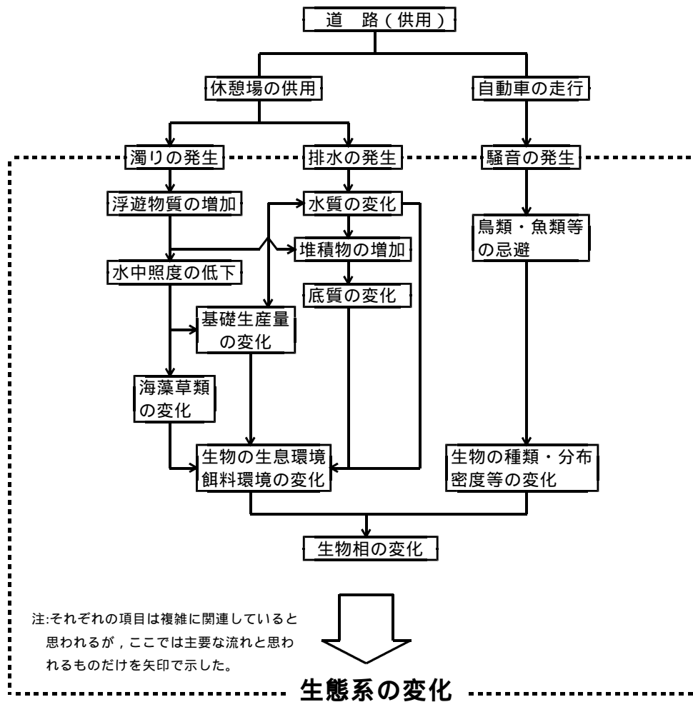
図 5 - 5 (3) 道路の供用に係る環境影響フロー
