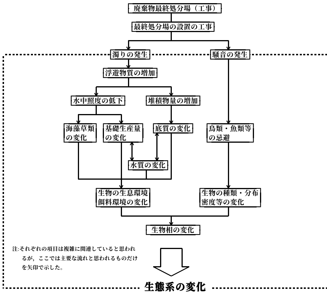
図5-4(1) 廃棄物最終処分場の工事に係る環境影響フロー
