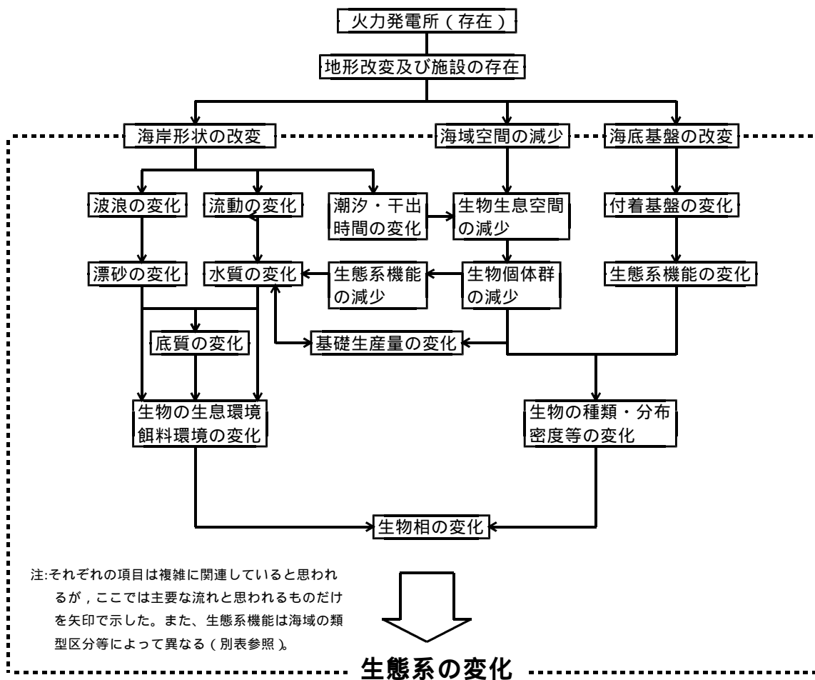
図 5 - 3 (2) 発電書（火力）の存在に係る環境影響フロー
