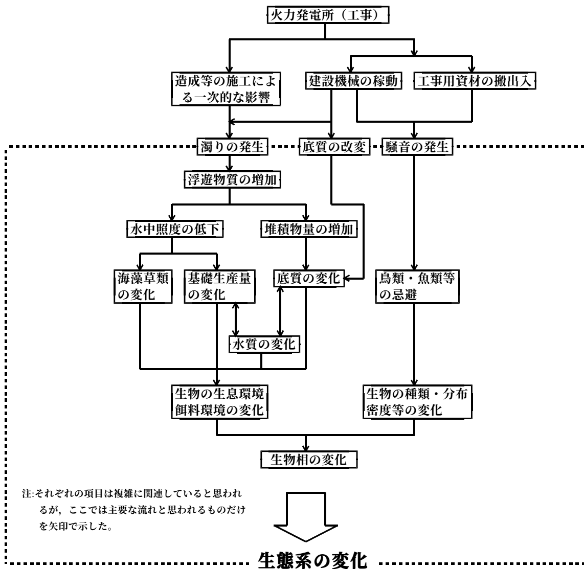
図5－3(1) 発電所（火力）の工事に係る環境影響フロー
